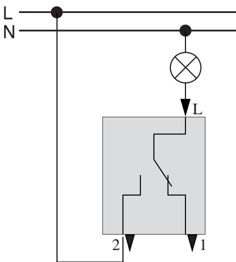
Aus/Wechselschalter Mxx3x16-0000
