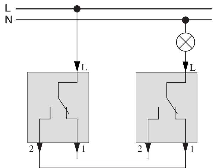
Aus/Wechselschalter Mxx3x16-0000
